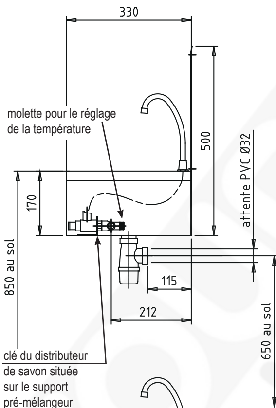
Lave-mains sans dossier, réf. 806 331
