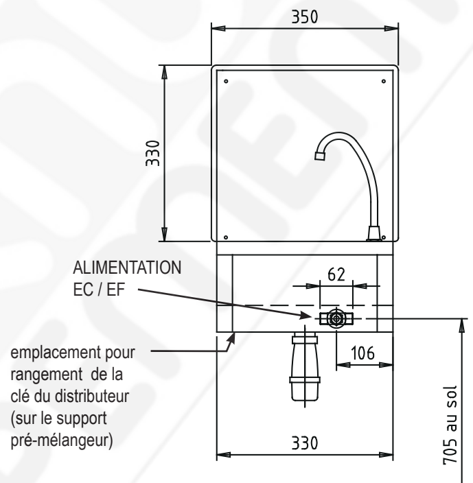
Lave-mains avec dossier et distributeur de savon, réf. 806 333
